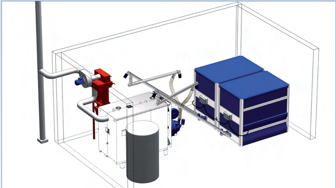
Variante mit zwei PelliStore™
