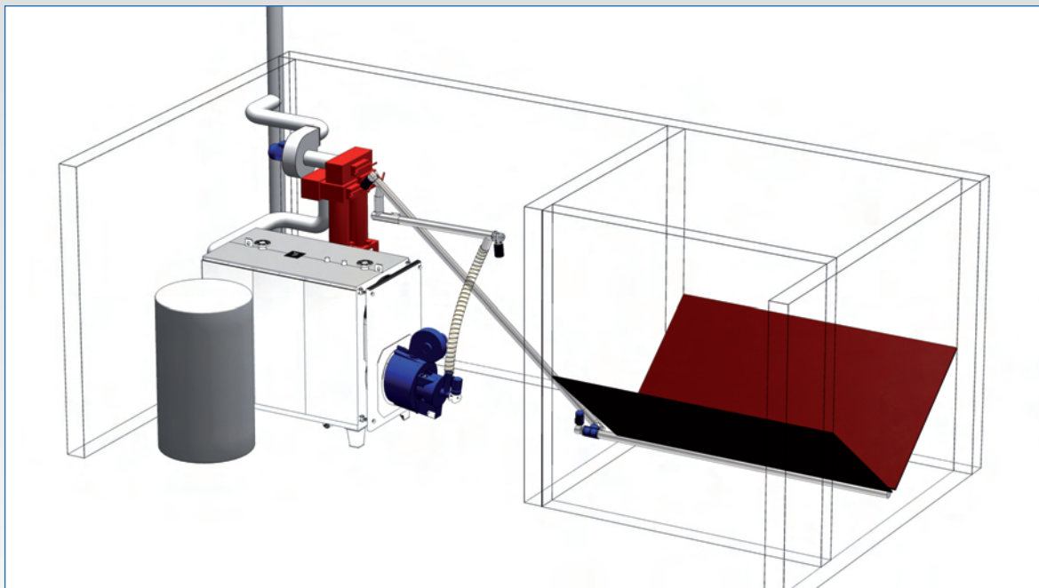
Pelletlager auf gleicher Ebene, ...
