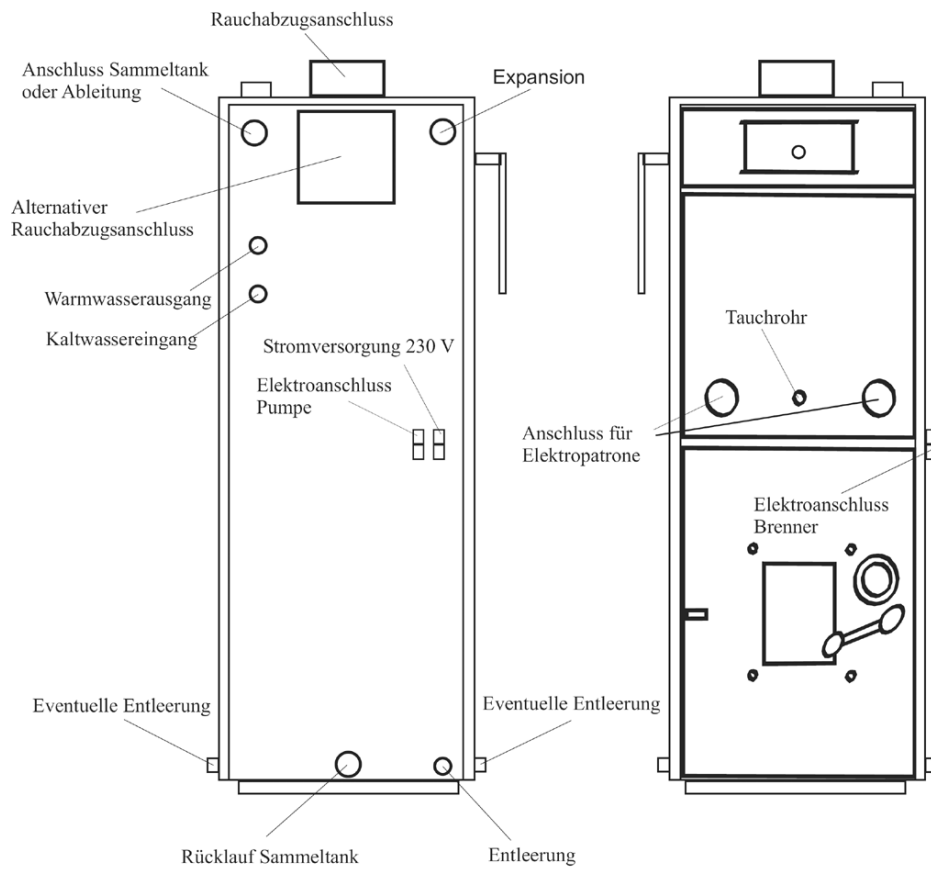
Anschlüsse intgral
